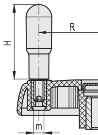
VDS...-K A-A
