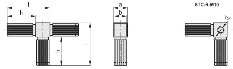
Na obrázku je vidět sestavený konektor. Tyto dva kusy mohou být sestaveny do různých tvarů v závislosti na rozměrech nebo provedení.
