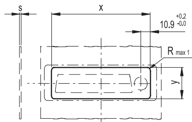
Vrtací šablona
