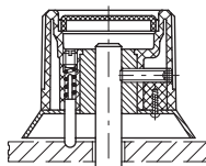
Sestava s upínacím šroubem a nastavitelným odpruženým šroubem
