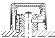
Sestava s upínacím šroubem, kuličkou a pružinou s nastavitelným tlakem
