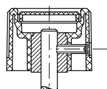
Sestava s upínacím šroubem
