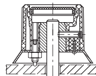
Sestava s upínacím šroubem a čepovým odpruženým šroubem s pojistnou maticí
