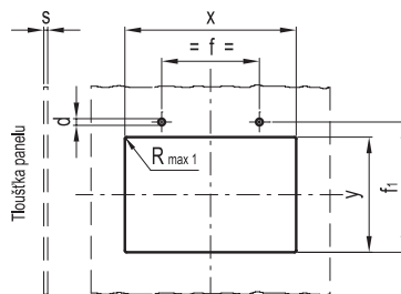
Výřezaný otvor (Před montáží madla obrušte hrany otvoru)
