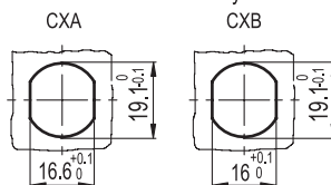
Montážní otvory
