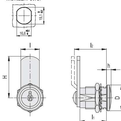
Montážní otvor
