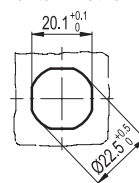
Montážní otvor
