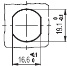
Montážní otvor
